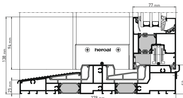
heroal S 77 HI, a 3 binari, sezione
